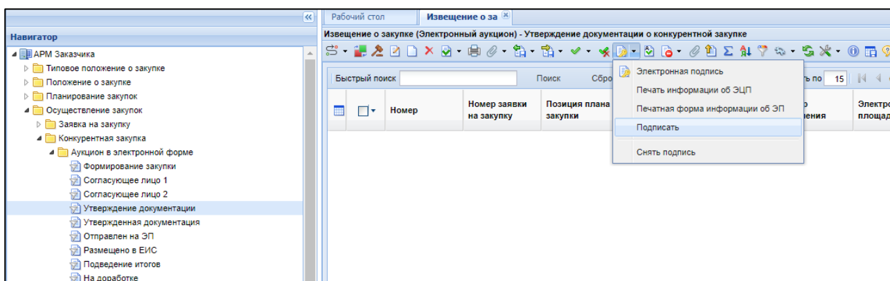
Рисунок 8. Утверждение документации
